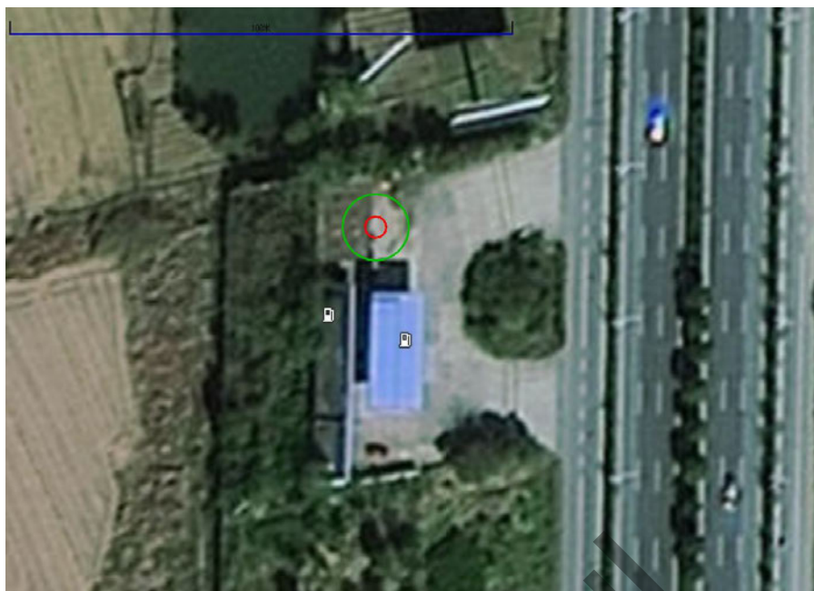
图 5-1 密闭卸油口小孔泄漏池火灾事故后果模拟图
