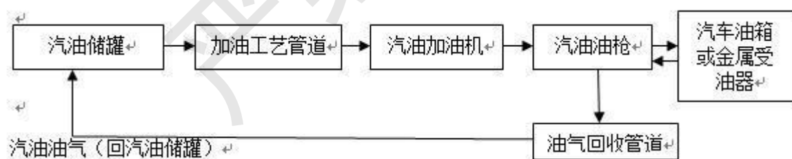
图 2-3 汽油加油及加油油气回收工艺流程图
