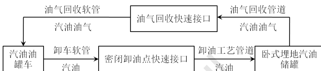
图2-1 卸油及卸油油气回收系统工艺流程图
